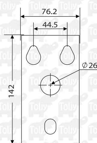
Contra Percha (Se coloca en el brazo)
