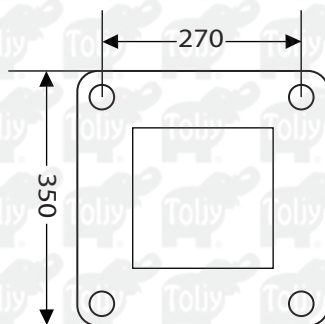
(350X350) 270 mm entre centros Para poste de 7 m a 9 m
