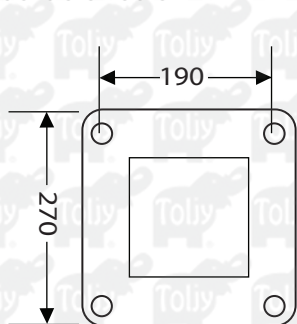
(270X270) 190 mm entre centros Para poste de 4 m a 6 m
